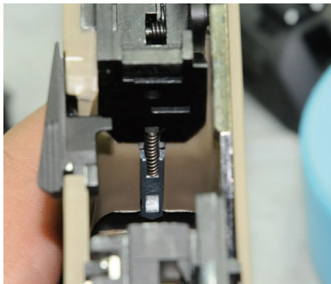
マガジンキャッチスプリング組込み方
